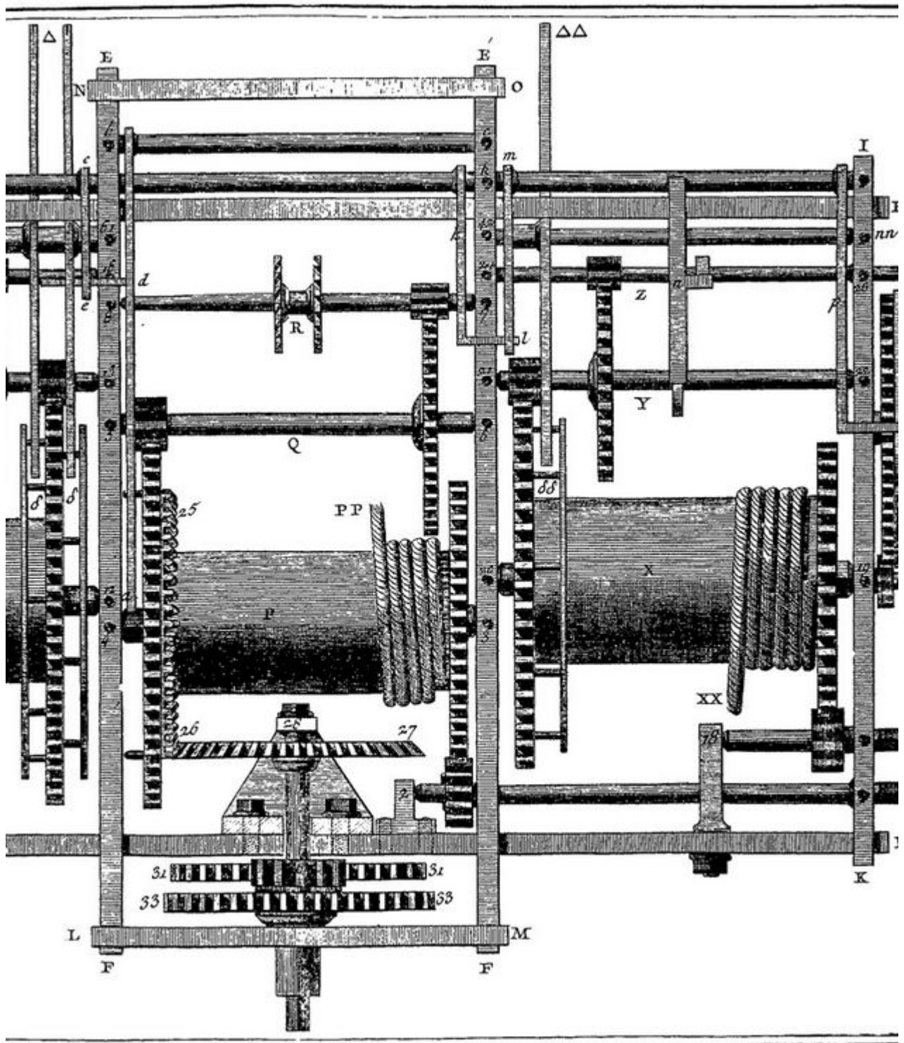
Horlogerie, Plan de l'Horloge Horizontale.
